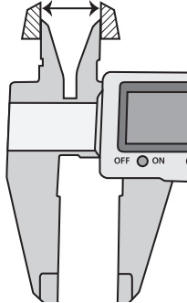
B. Sisämittaus
